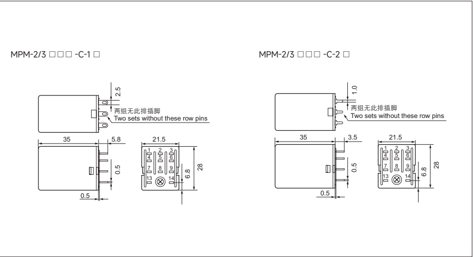
外形尺寸 PROFILE DIMENSION
